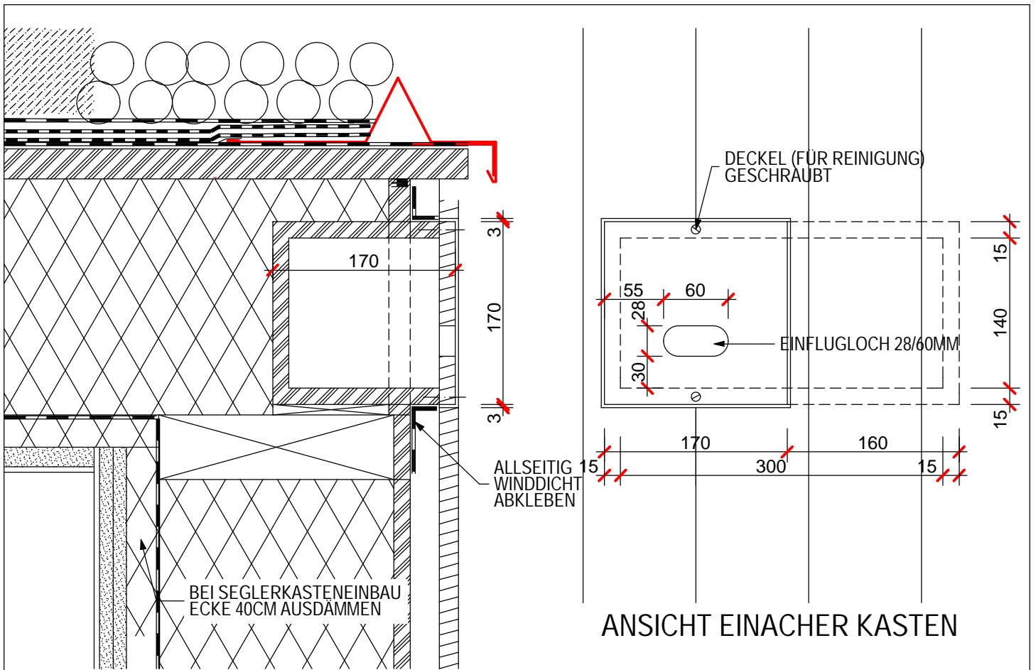
ORT+TRAUFDDETAIL MIT SEGLERKASTENEINBAU
