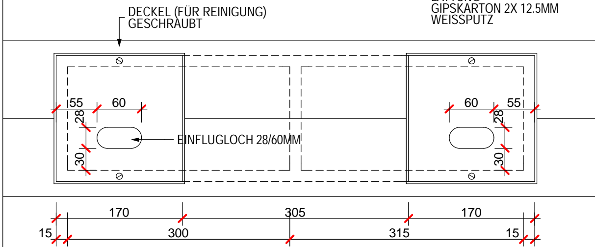
ANSICHT DOPPELKASTEN
